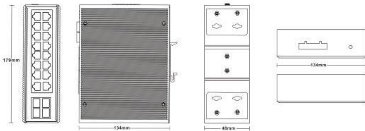
尺寸图
