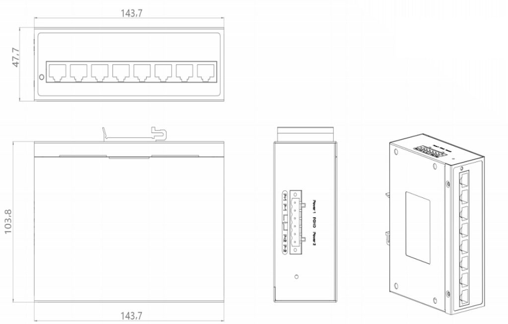
ISE5008D 尺寸
