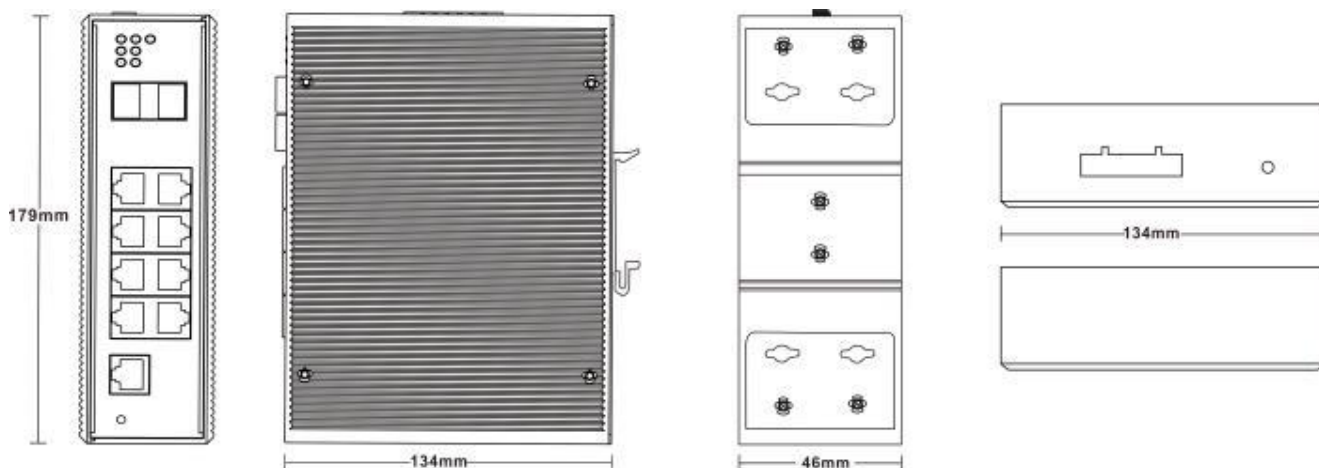
ISM3010D-S 尺寸
