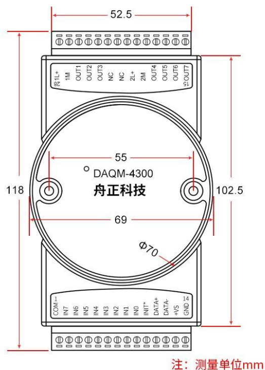
正视图
