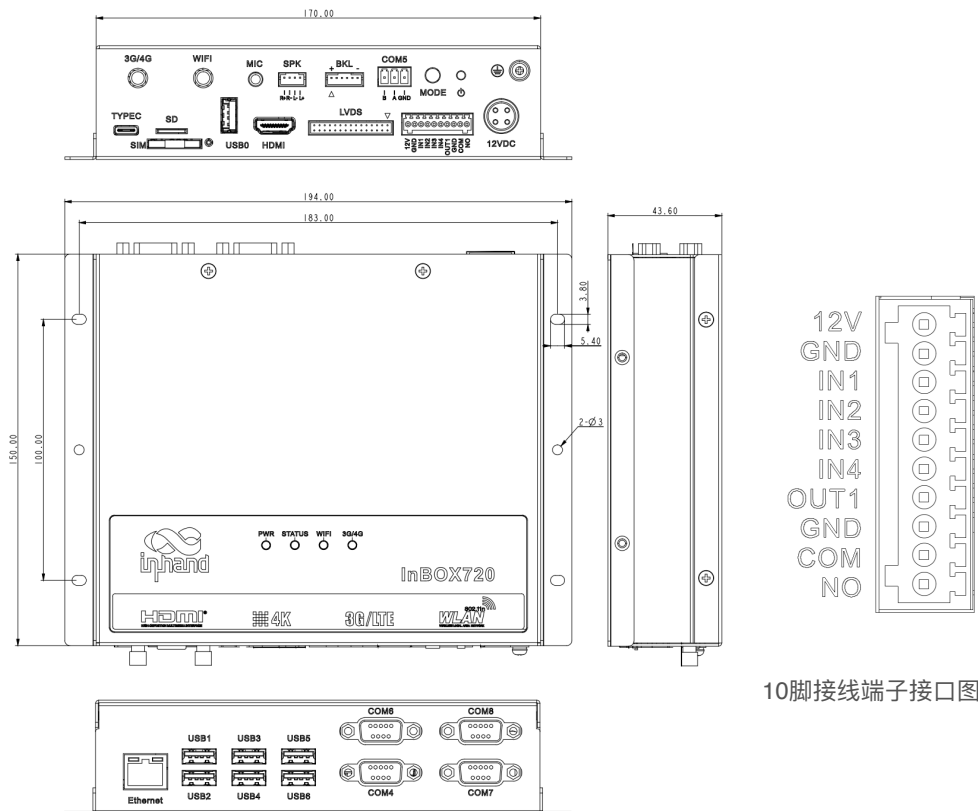
InBOX720产品尺寸图
